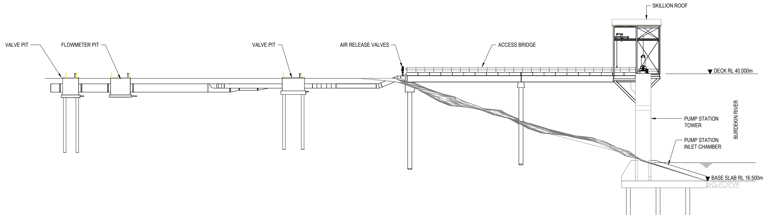
SITE SECTION SCALE 1:250
