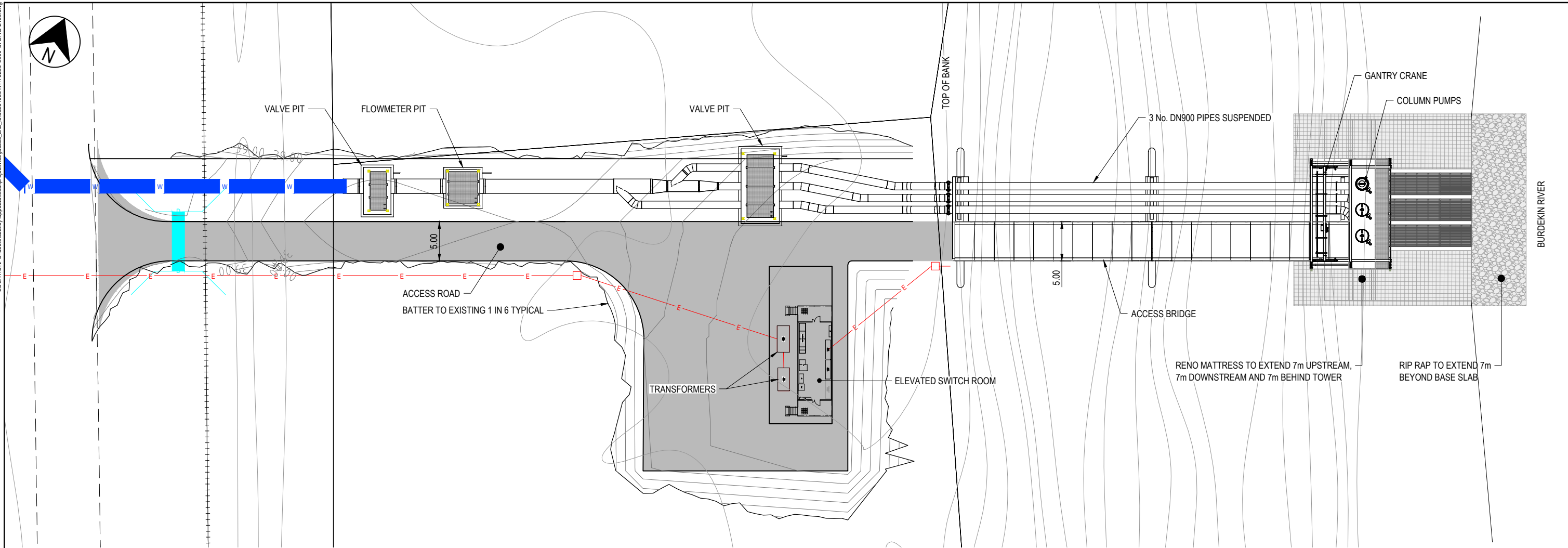
SITE PLAN SCALE 1:250
